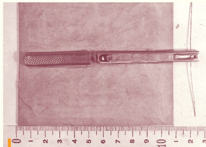
Esta foto mostra um conjunto de disparo ainda sem desativação, ao ser retirado do envelope. Dentro do recipiente ficou o explosivo plástico "C3", envolvido por um papel tipo 'mata-borrão', porque soltava uma espécie de óleo. O último invólucro contém fulminato de mercúrio que, se explodir, pode arrancar o dedo de alguém.
