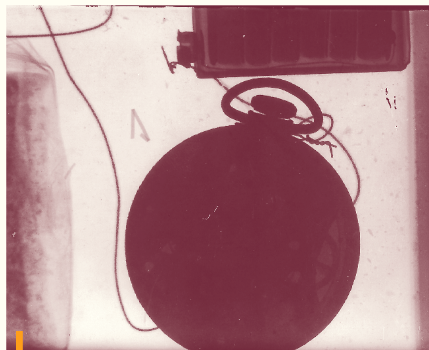
Raio-X de uma bomba relógio montada.
