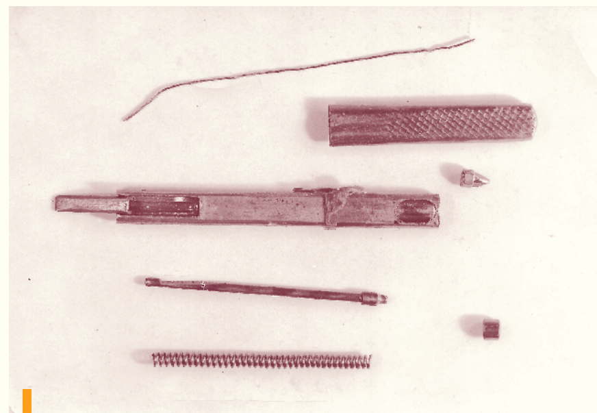
Conjunto de peças, componentes do sistema que faz funcionar o disparo de explosivos.
